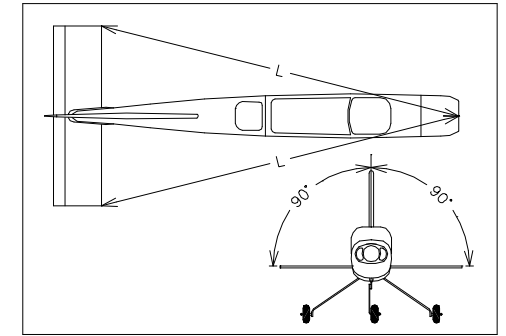
FIGUA 4 – instalação do trem de pouso
