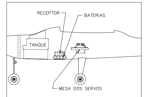
FIGURA 5 – instalação receptor e baterias
