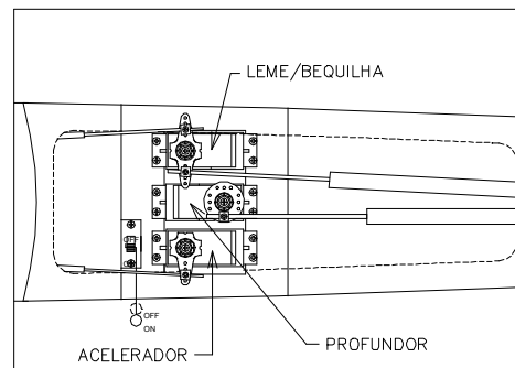
FIGURA 2 – mesa de servos
