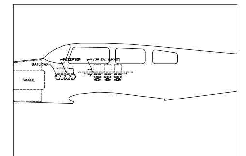
FIGURA 5 – instalação receptor e baterias
