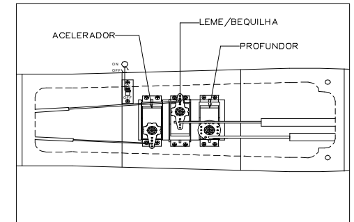
FIGURA 3 – instalação do estabilizador
