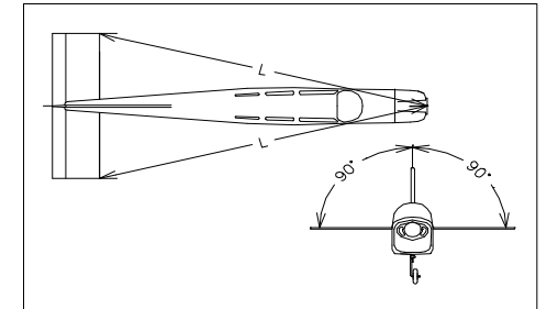
FIGURA 4 – instalação do trem de pouso
